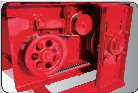
Vis d'alimentation avec un arbre de 2" supporté par deux coussinets à cage de fonte. Des protecteurs sur charnières facilitent l'accès à tous les mécanismes.
